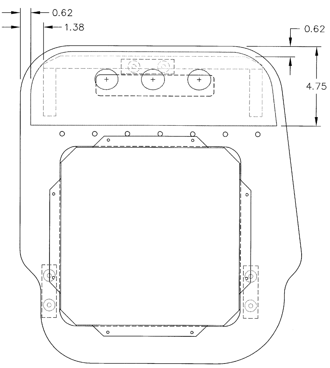
MGA SEAT BASE ASSEMBLY, LH
