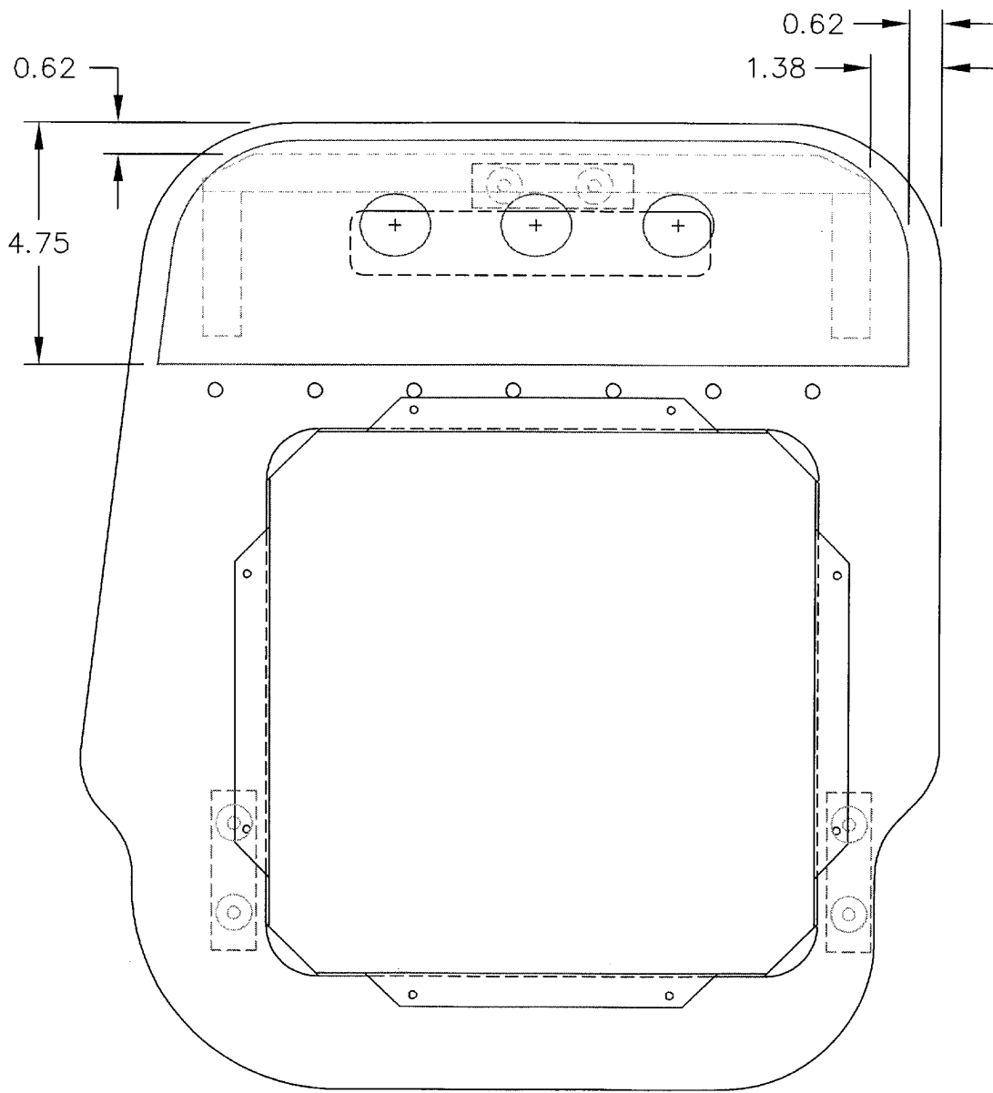
MGA SEAT BASE ASSEMBLY, RH
